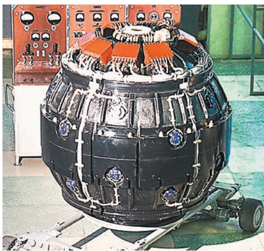
Атомный заряд бомбы РДС-1.
