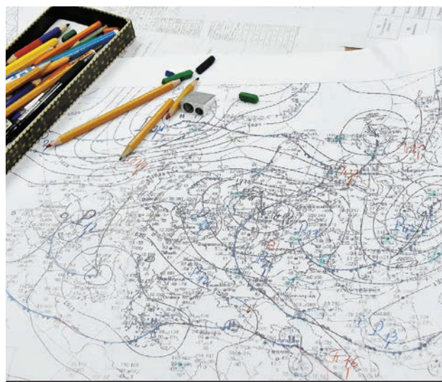
Так выглядит синоптическая карта.
